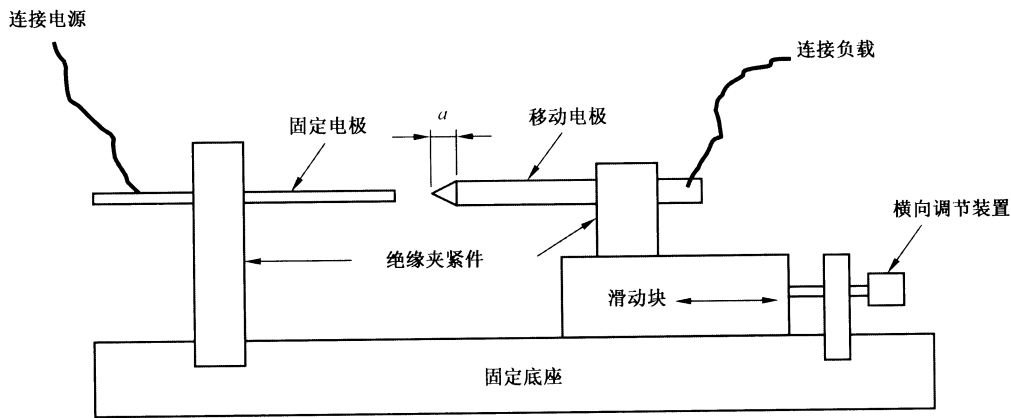
图 5 电弧发生器
