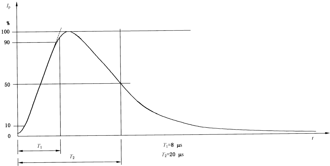
图 31 8/20 μs 浪涌电流脉冲
