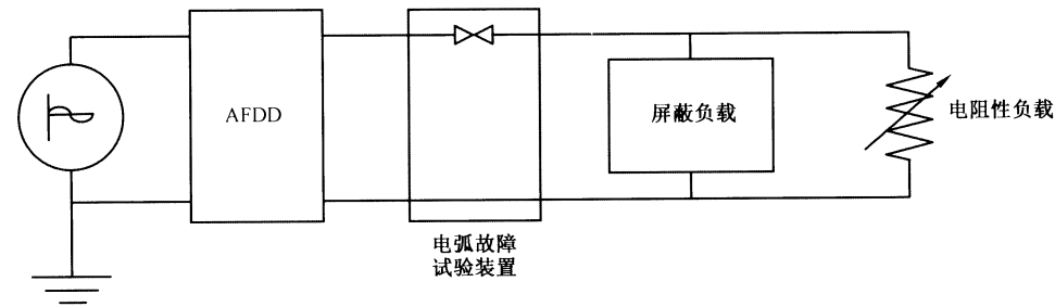
图 11 屏蔽试验的试验配置
