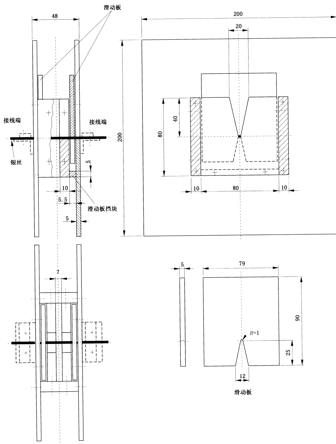
图 K.1 验证 AFDD 所能承受的最小 I^2t 和 I_p 值的试验装置
