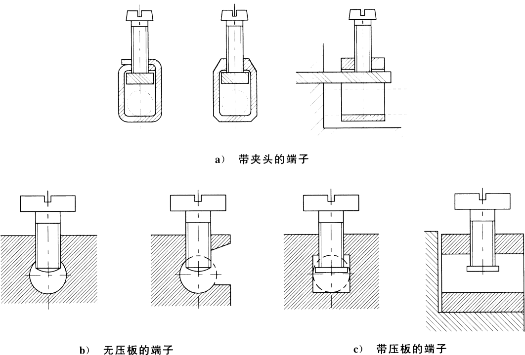
图 H.1 柱式端子示例
