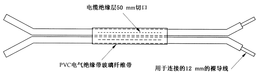
图 36 电缆试品的准备(9.9.2.6)
