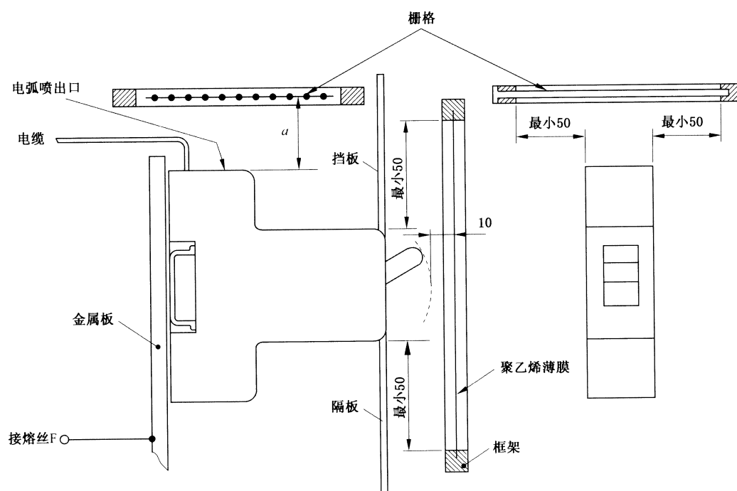
图 C.1 试验装置
